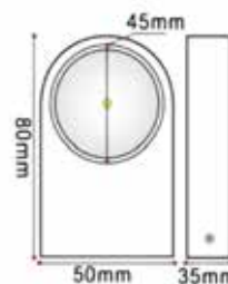
Maßskizze Beam 2
